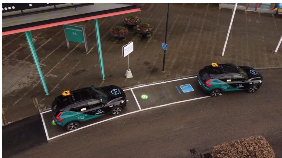
Rys. 22 Przykład testowania ładowarek indukcyjnych firmy Momentum Dynamics w Szwecji – moc ładowania ponad 40 kW
